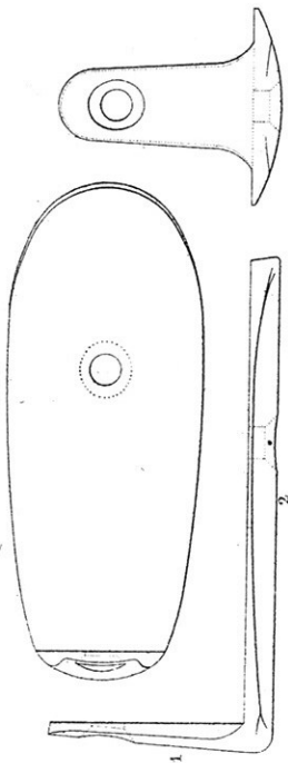
Fig 6 _Plaque de couche des fusils.
