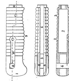
Fig. 6. Poignée.
