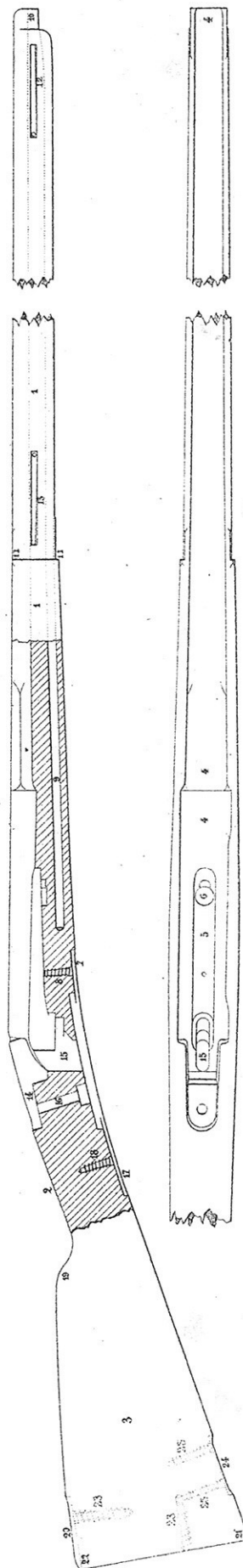
Fig. 3. Monture de la Carabine de Gendarmerie M le 1874.
