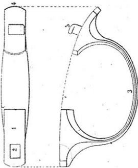
Fig. 20. Pontet.
