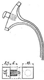
Fig 10.- Pontet du Revolver M e 1873 Remplacem nt du T
