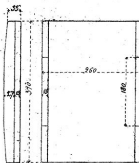
Planchette de pression.
