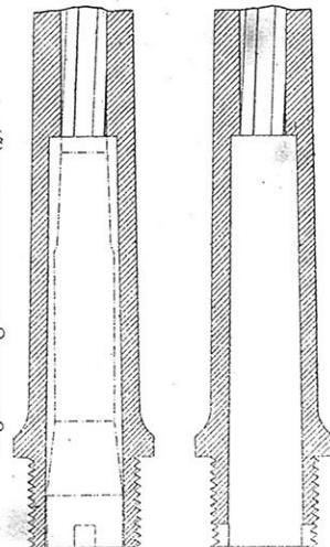
Fig. 20. _Logement du Tube ( \frac{1}{2} ).
