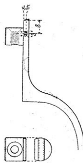
Fig 3.-Pontet du Fusil M e 1874.
