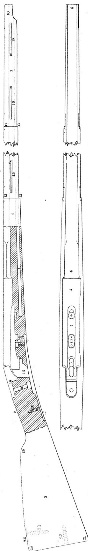
Fig. 1..Monture de la Carabine de Cavalerie M re 1874.
