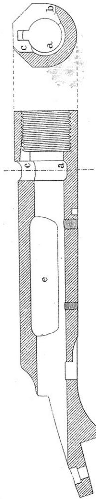
Fig 2. — Tête mobile.
