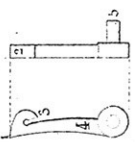
Fig. 14. Ressort de détente.
