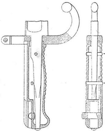
Fig. 10. Coupe longitudinale de la monture.
