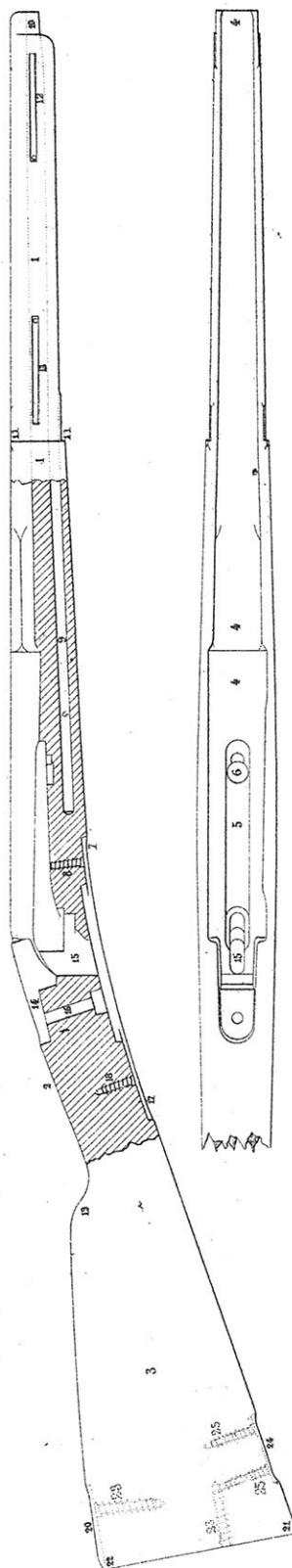
Fig. 3. Monture du Mousqueton. M le 1874.
