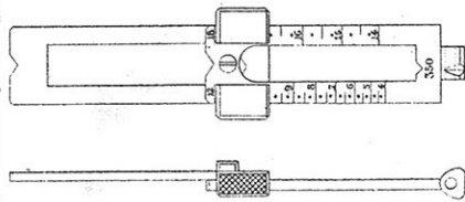
Fig 1. Assemblage de la planche mobile et du curseur à rallonge.
