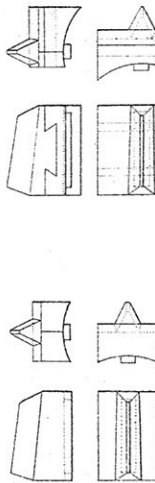
Guidons des Mousquetons. ( \frac{1}{4} ). Fig. 15. M le 1874.
