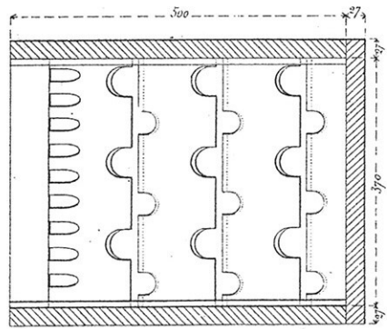
Coupe suivant CD. ( \frac{1}{10} ).
