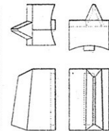
Guidons des Carabines. ( \frac{1}{4} ). Fig. 13. Gendarmerie M le 1874.
