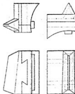
Guidons des Mousquetons. ( \frac{1}{4} ). Fig. 15. M le 1874.
