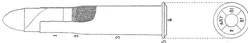
Fig. 1. Cartouche à balle. ( \frac{1}{4} ).
