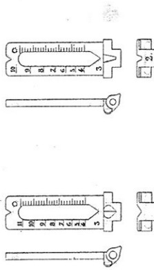
Fig 23. Carabines M le 1874.
