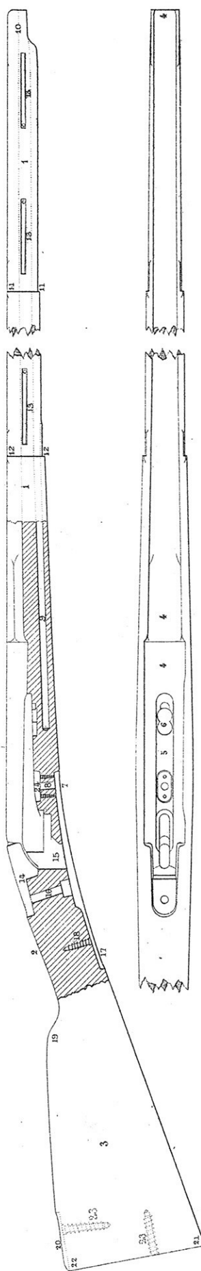
Fig.2. Monture de la Carabine M c 1866-74.
