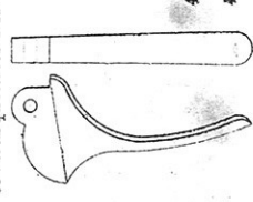
Fig. 12. Détente du Fusil M e 1874
