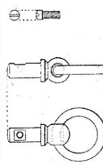
Fig. 8. Anneau de calotte. Pivot d'anneau de calotte et sa vis
