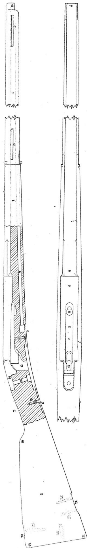
Fig. 1. Monture du Fusil M le 1874.
