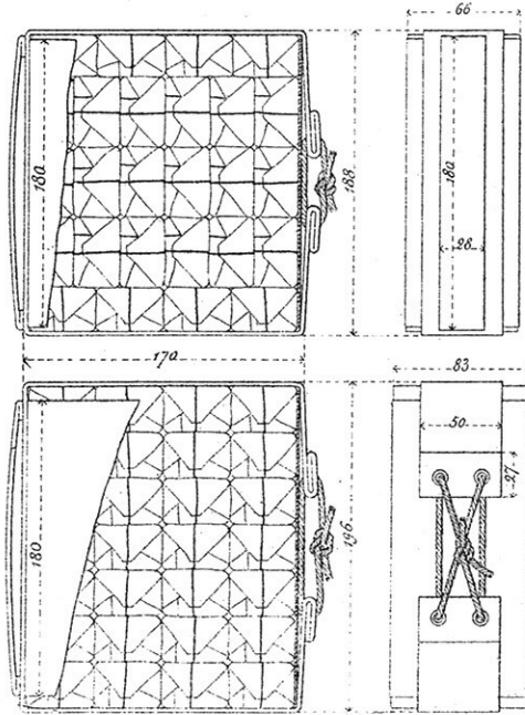
Caisse blanche pour cartouches à balle M e 1873.
