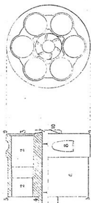
Fig. 1. Barillet.
