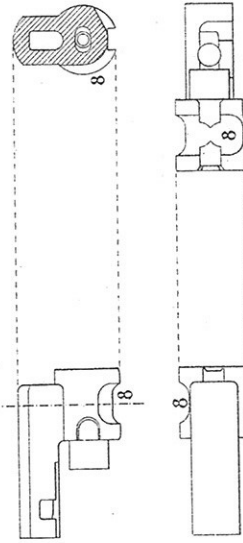
Fig 2. — Tête mobile.
